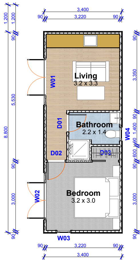
Floor Plan Wall Setout 1:100
